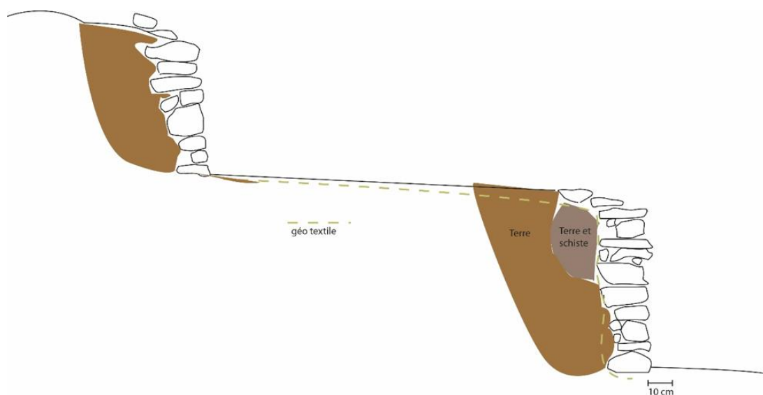
Fig. 03 : Vue en coupe des murs avant restauration.
