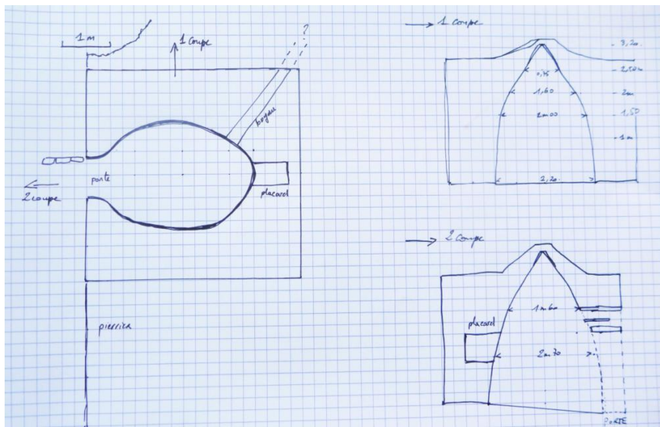
Plan et coupes
