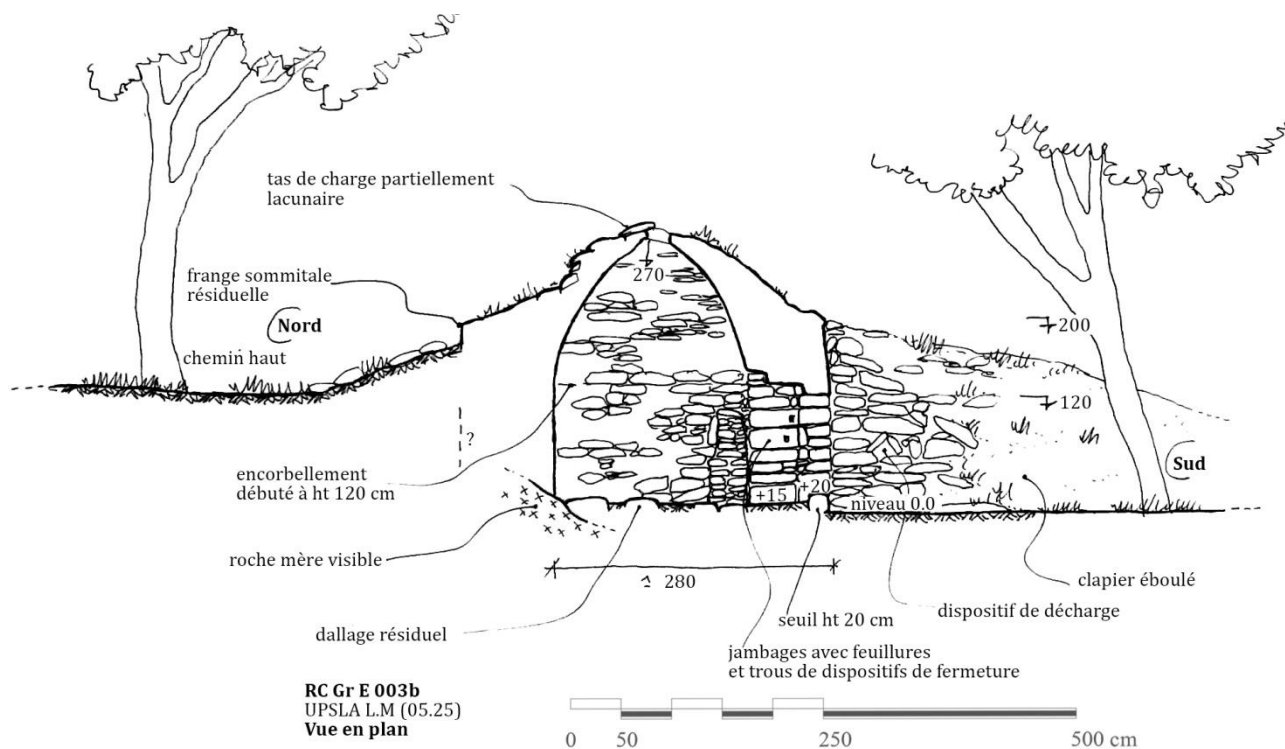
Fig. 11 : Vue en coupe AA' (UPSLA)
