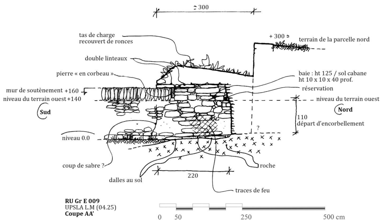
Fig. 08 : Vue en coupe
