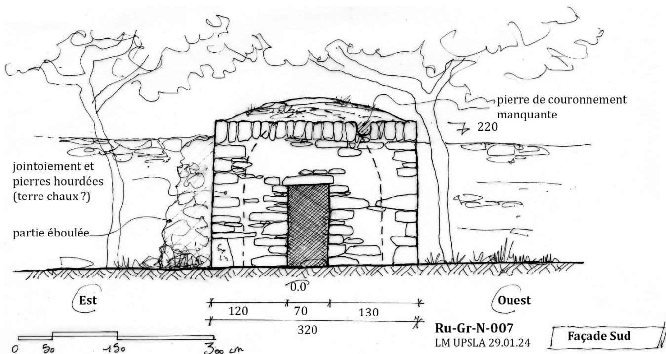
Fig. 08 : vue de la façade Sud
