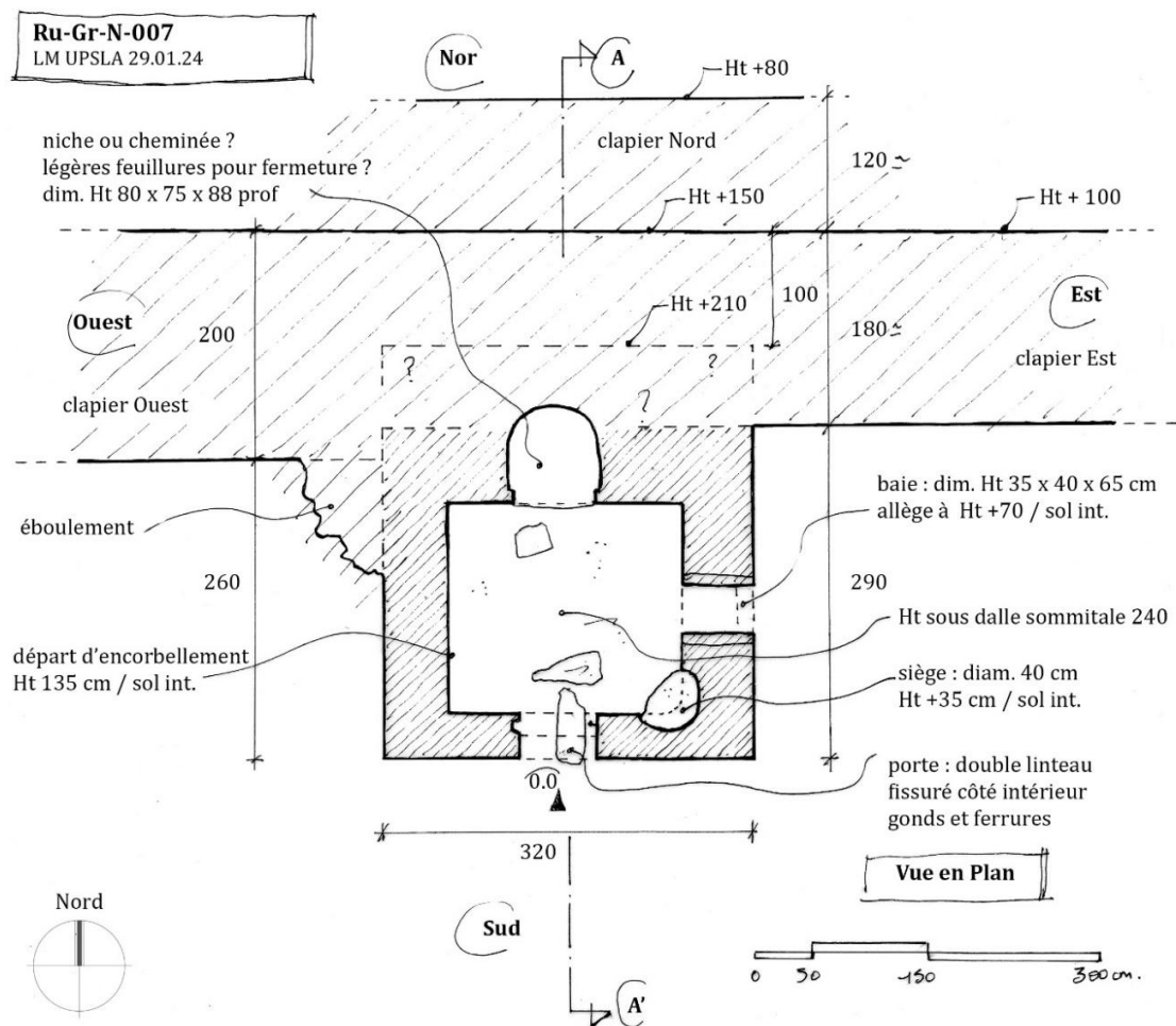
Fig. 06 : vue en plan
