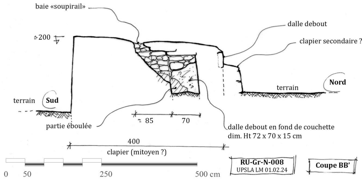
Fig. 09 : Coupe BB'
