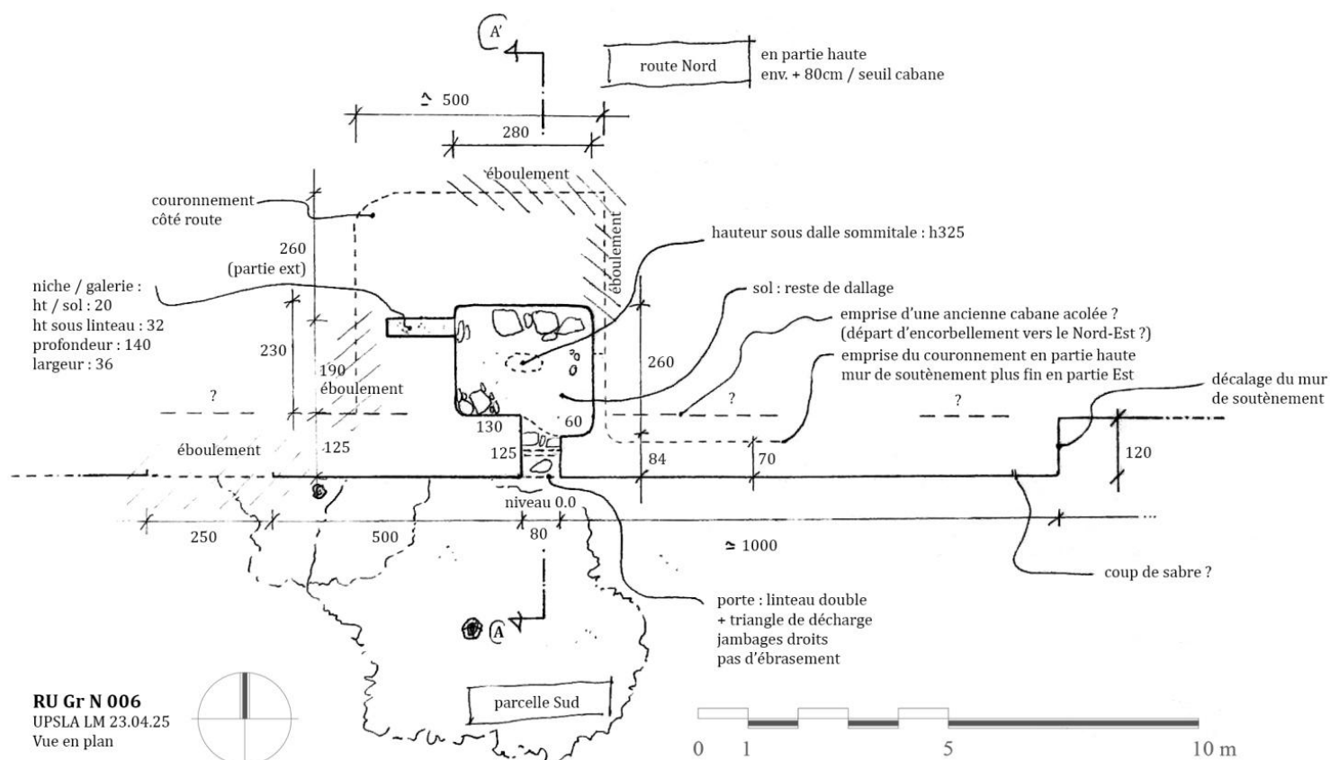
Fig. 08 : Vue en plan
