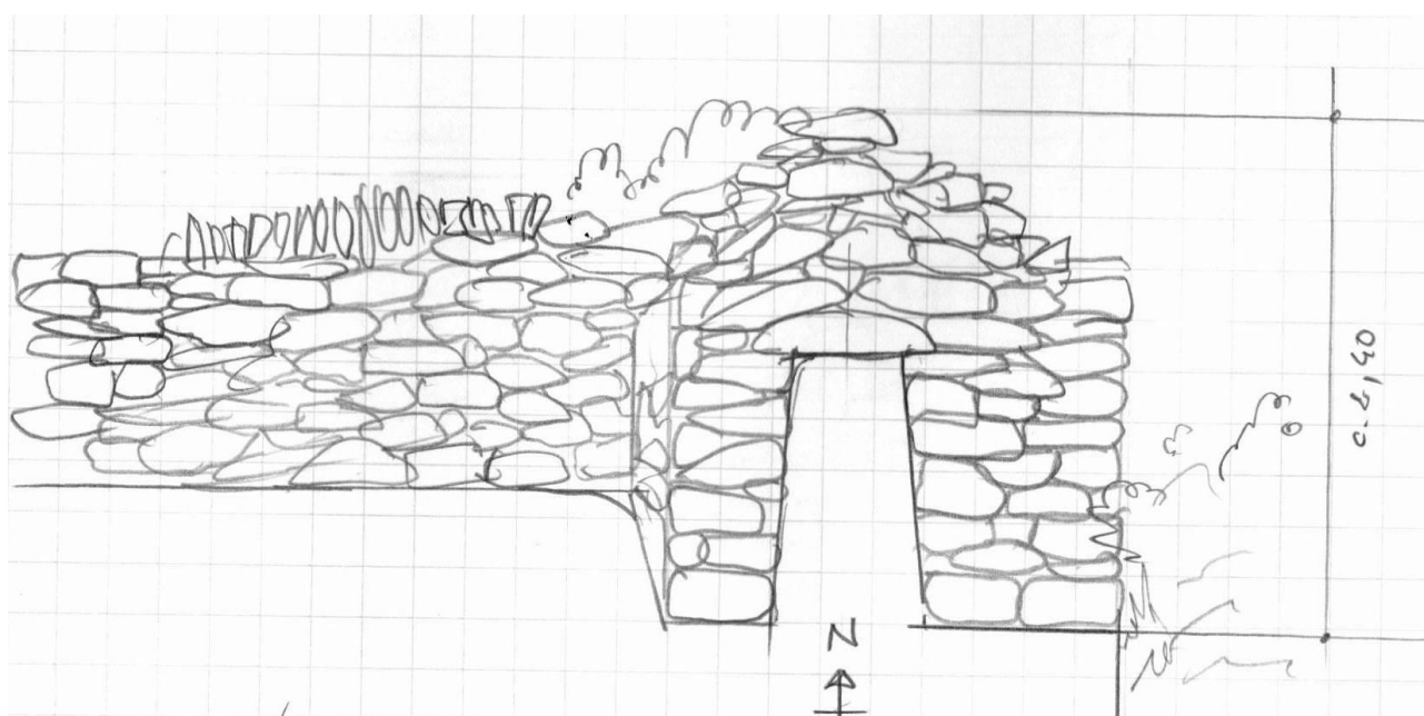
Elévation Sud
