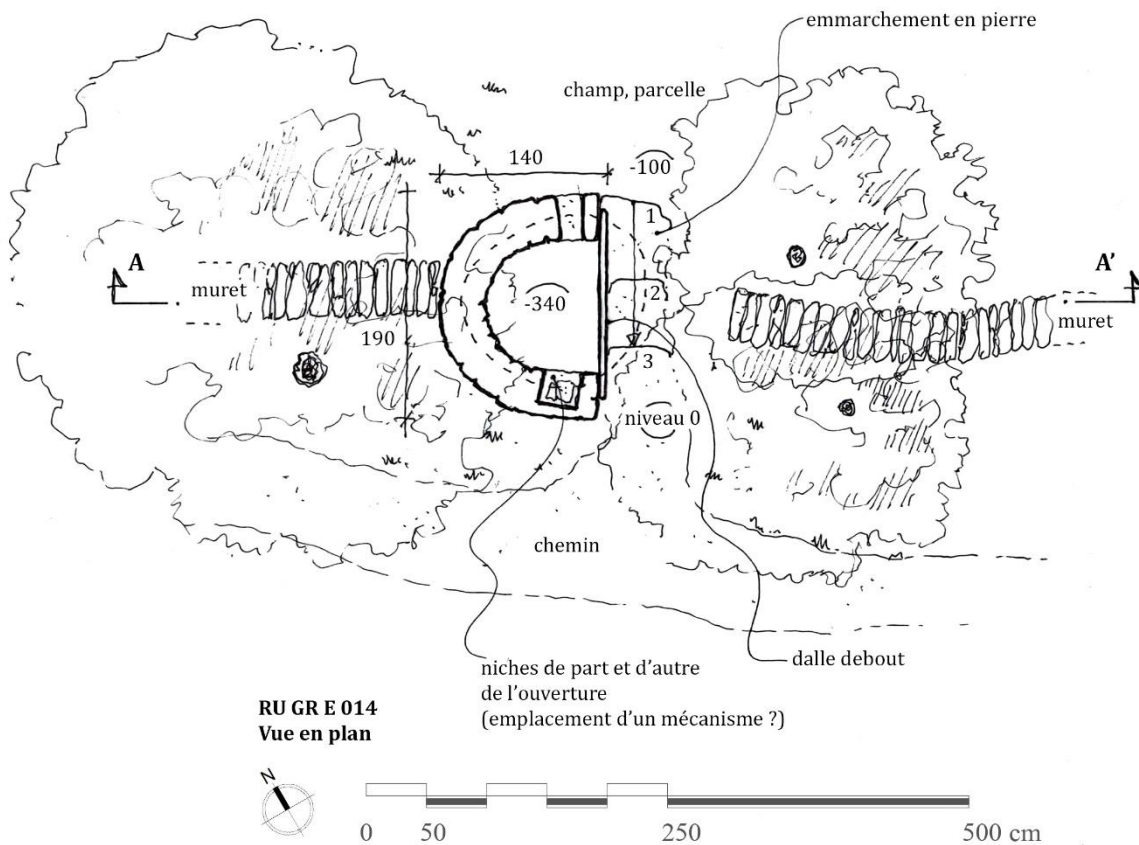
Fig. 06 : Vue plan
