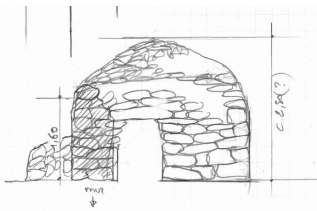
Elévation Ouest
