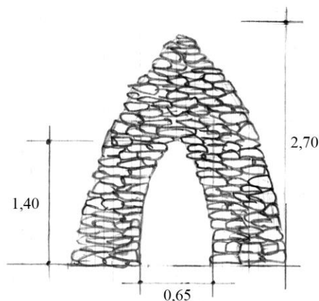
Cabane 2 Elévation intérieure Est Détail du passage vers la seconde cellule
