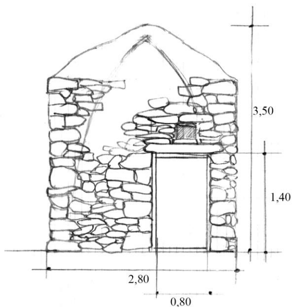
Cabane 2 Elévation Est Détail de la porte d'entrée
