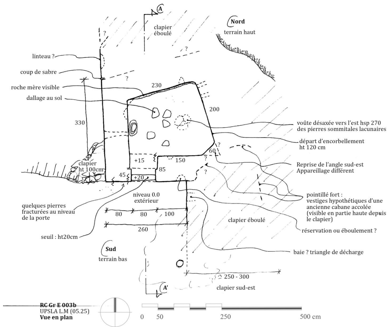
Fig. 09 : Vue en plan (UPSLA)
