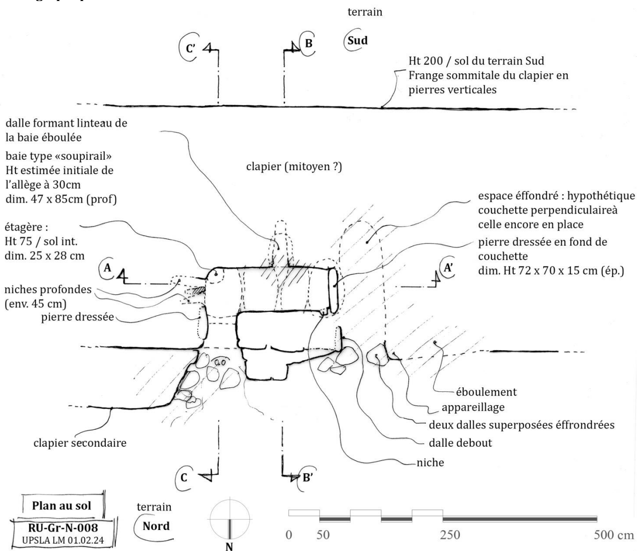
Fig. 06 : plan au sol
