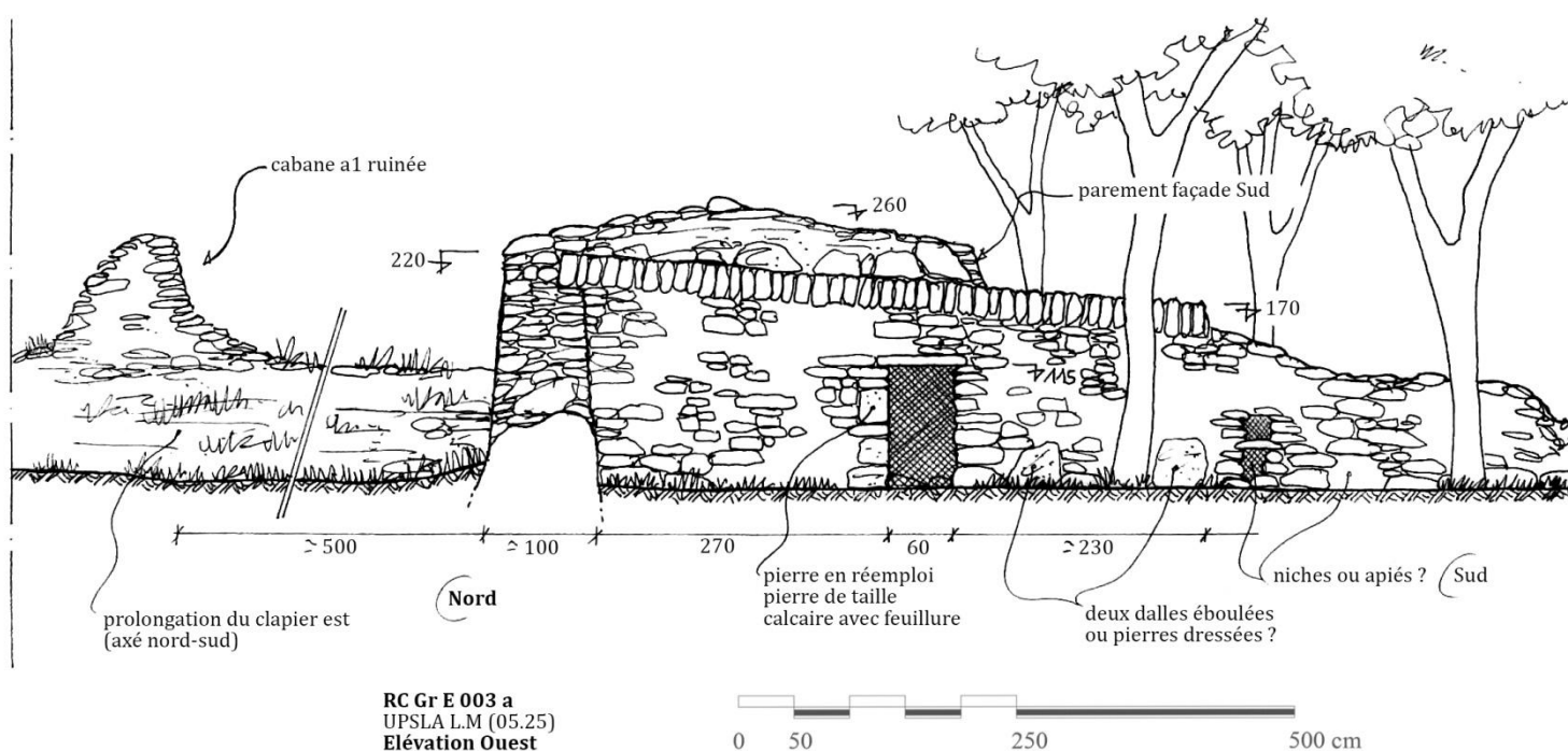
Fig. 08 : Elévation Ouest
