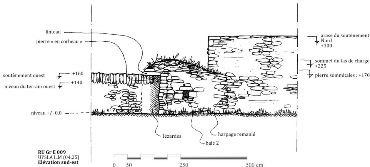
Fig. 07 : Elévation sud-est
