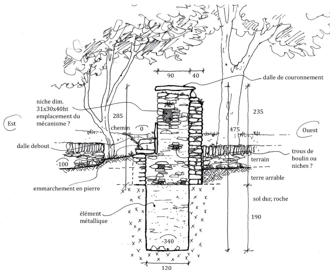
RU GR E 014 Coupe AA'
