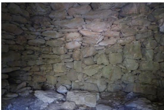
Fig. 05 : mur int. nord, granulométrie variable, dallage, niche. / Fig. 06 : niche / galerie en partie int. ouest.
