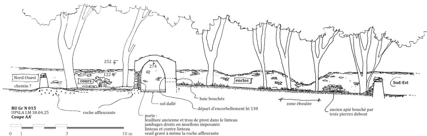
Fig. 07 : Coupe AA'
