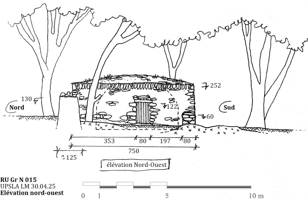
Fig. 08 : Elévation nord-ouest
