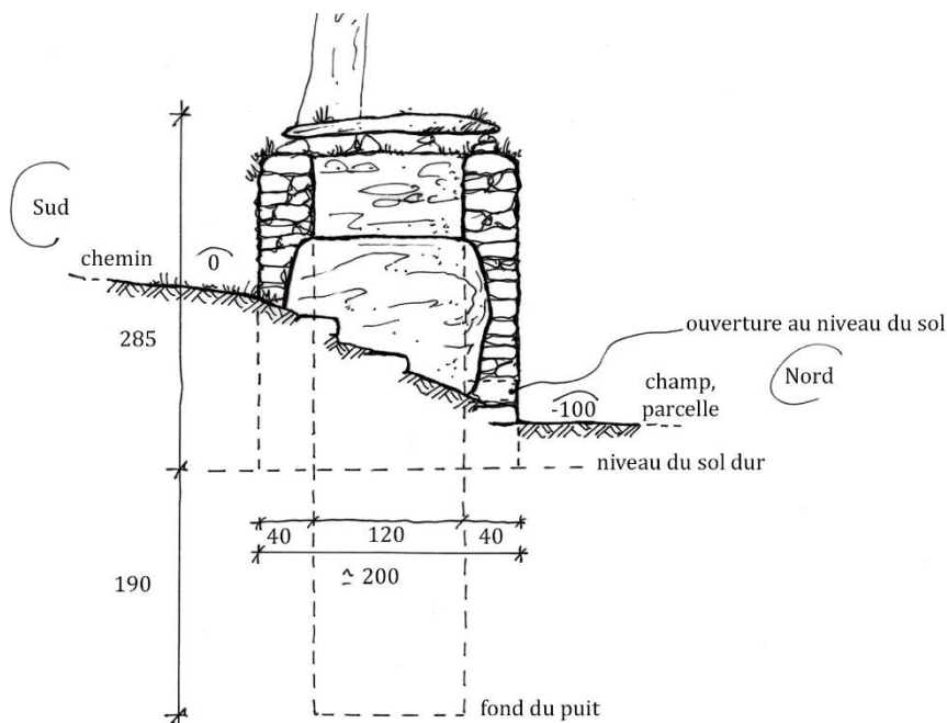
RU GR E 014 Élévation Sud
