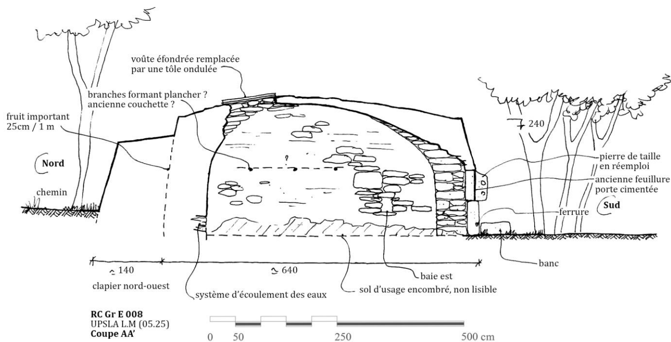
Fig. 10 : Coupe AA'
