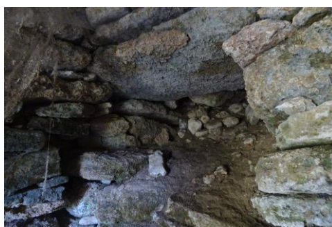
éboulement de la niche et vue du drain du mur de soutènement arrière
