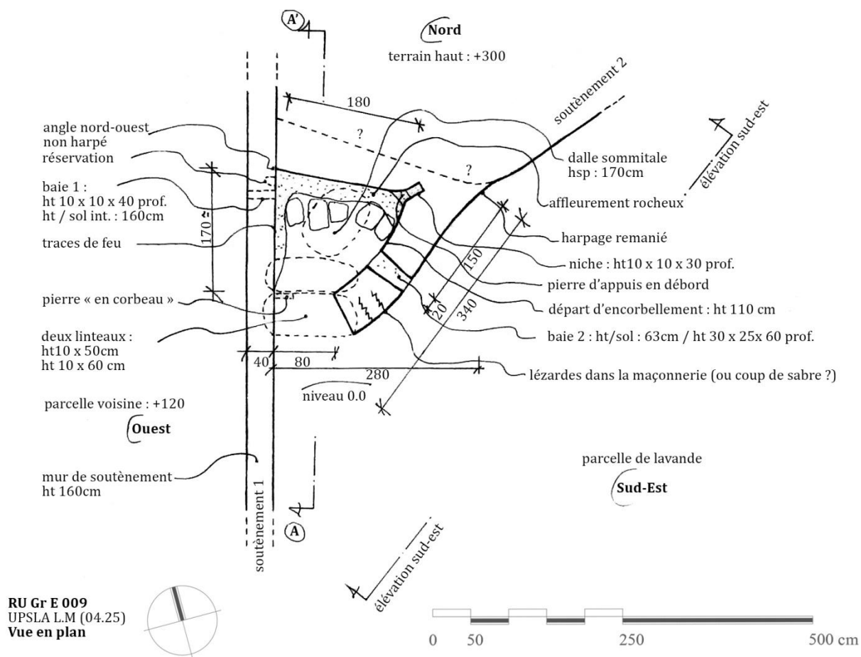
Fig. 06 : Vue en plan
