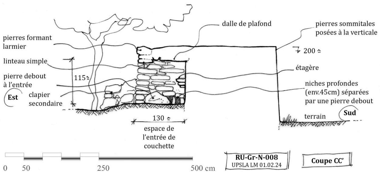
Fig. 10 : Coupe CC'
