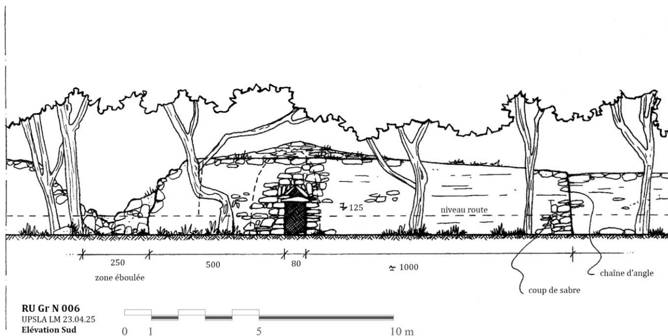
Fig. 09 : Elévation Sud
