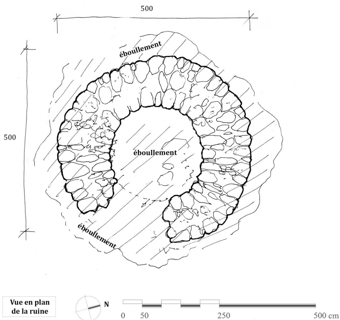
Emprise du départ d'encorbellement
