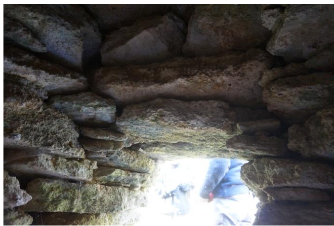
Lindeau intérieur et départ d'encorbellement
