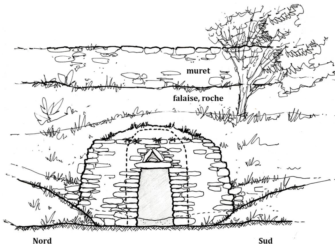
Elévation Ouest
