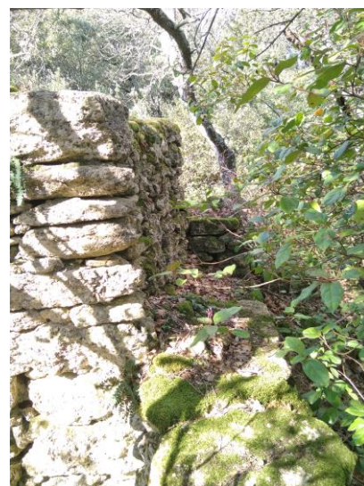
Banquette formée sur le clapier
