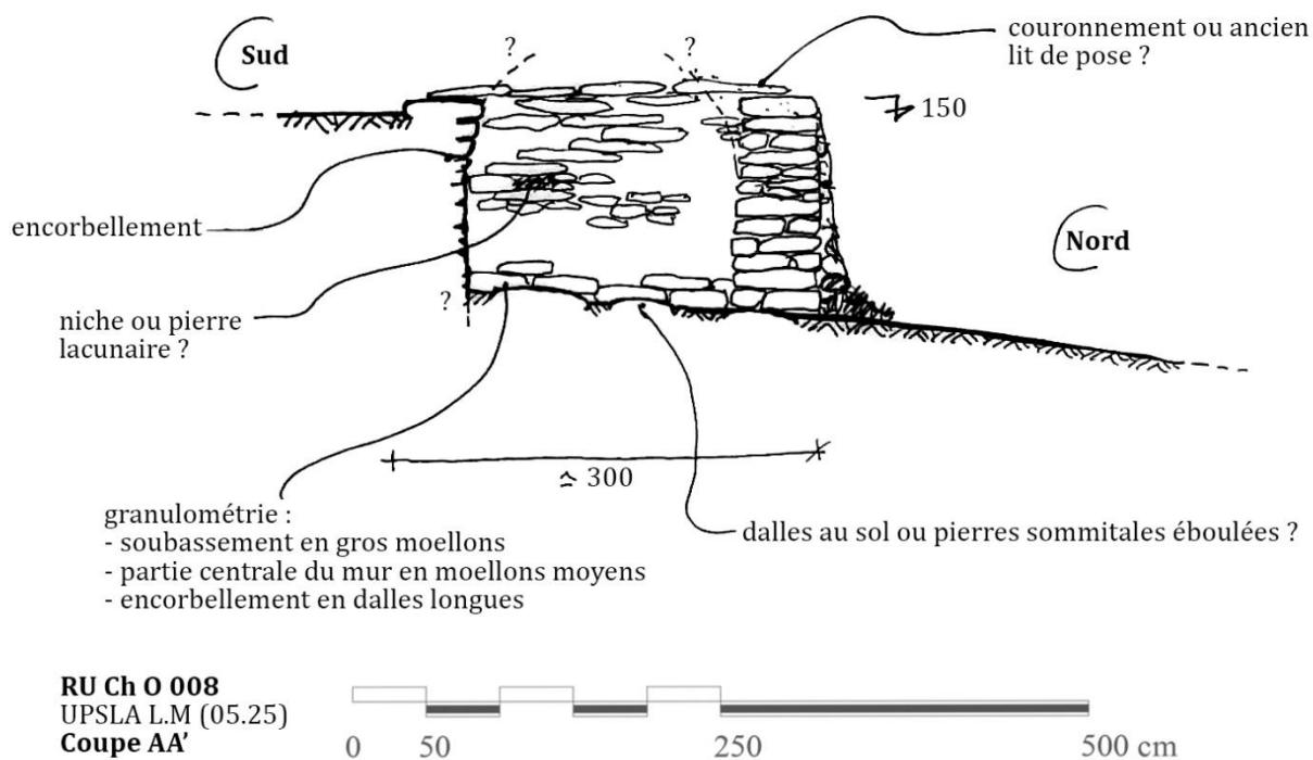
Fig. 08 : Coupe AA'
