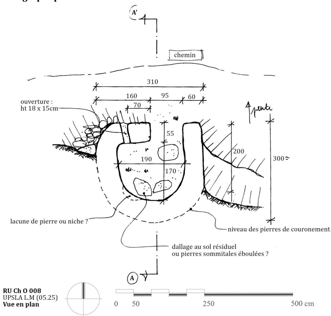
Fig. 06 : Vue en plan
