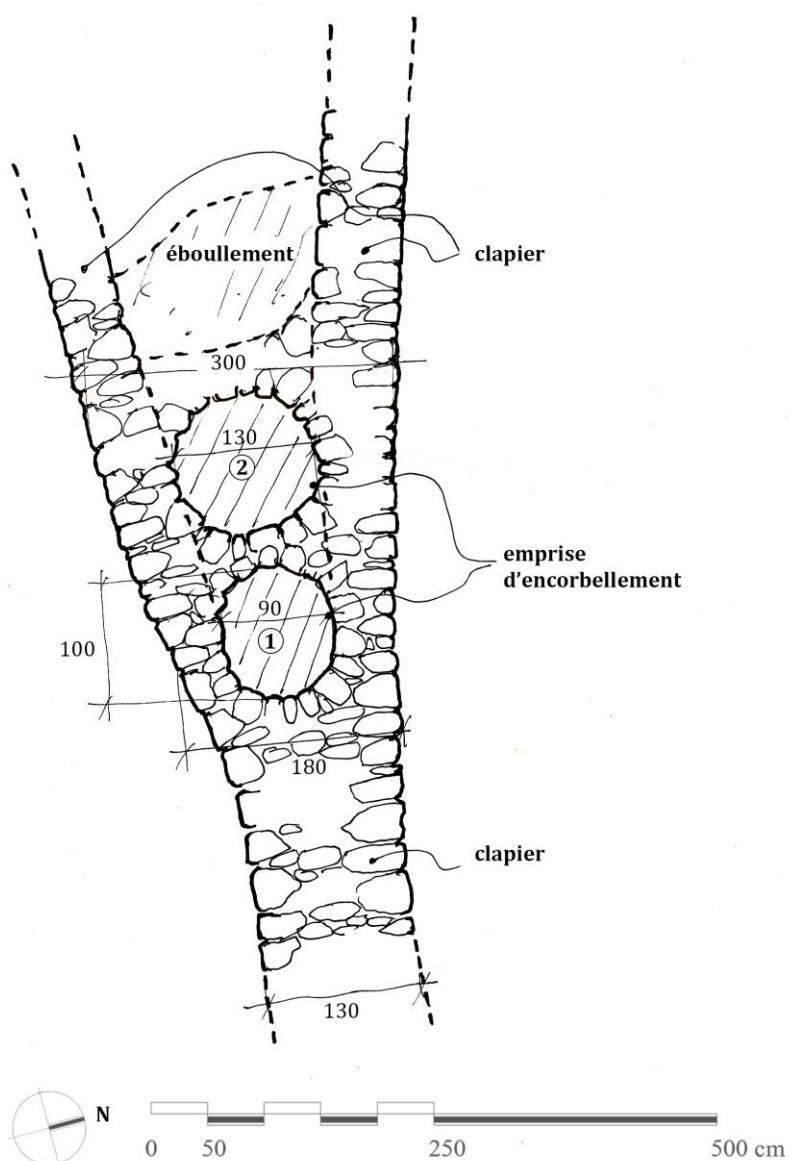
Mur de clôture contre lequel la cabane s'adosse
