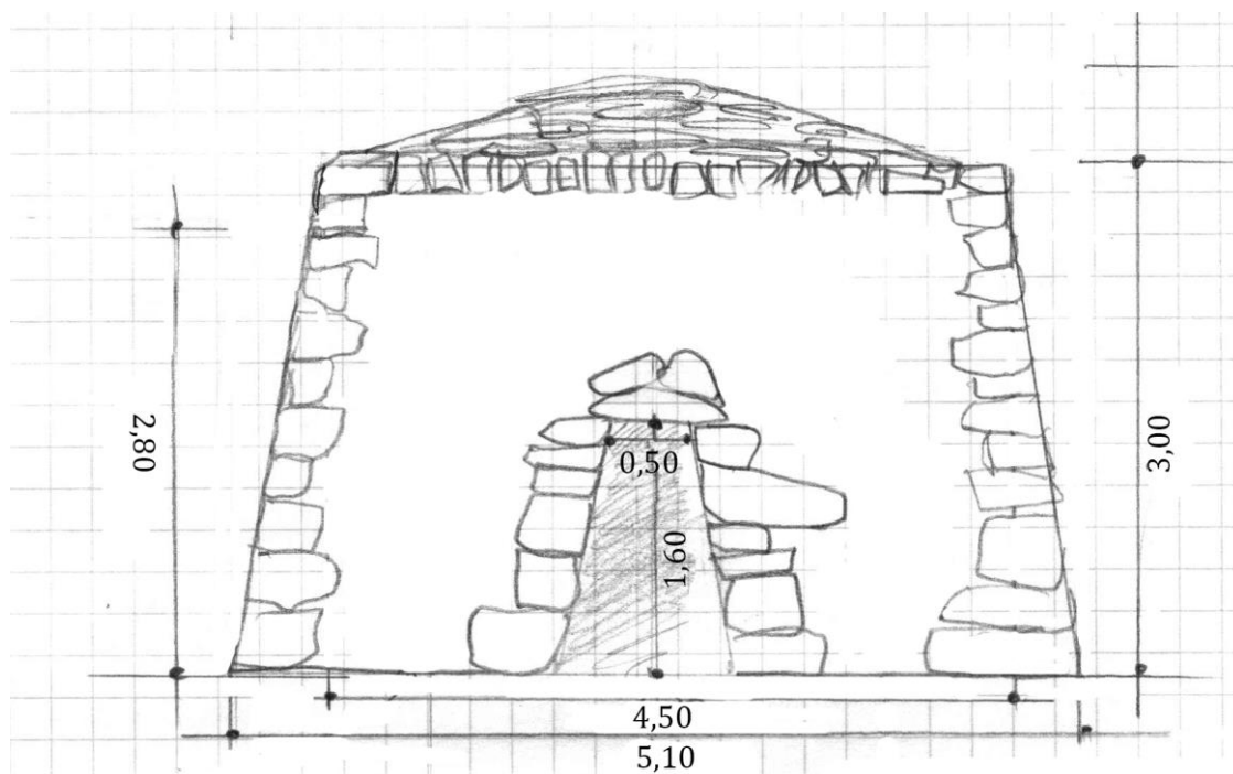
Elévation Sud
