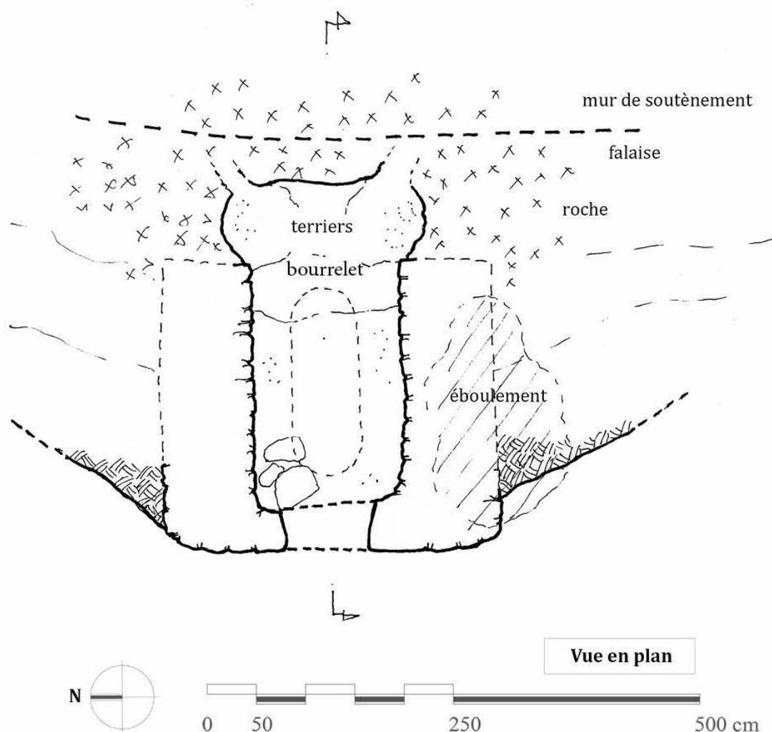
Terriers en creusés par des animaux en fond de cabane
