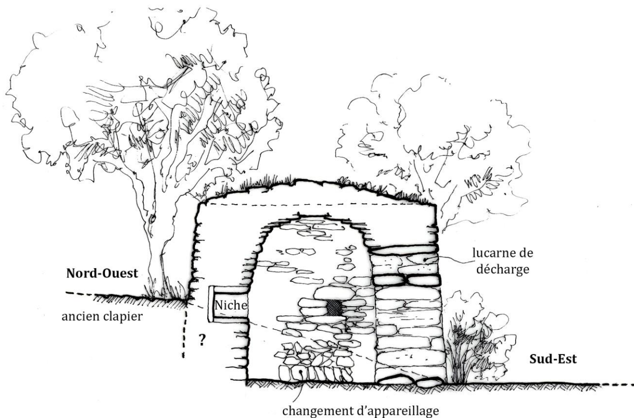
Coupe transversale
