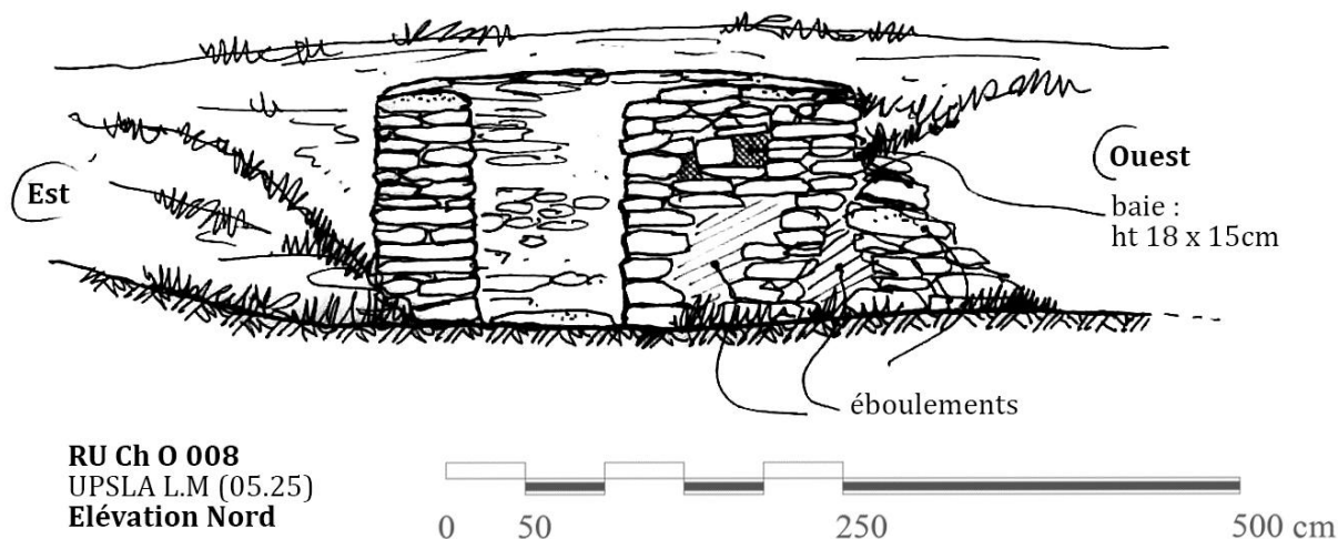
Fig. 07 : Elévation Nord
