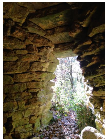
Encorbellement de la porte
